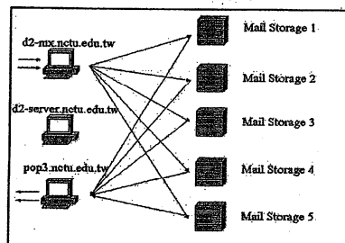
圖一 交大分散式電子郵件系統架構圖
